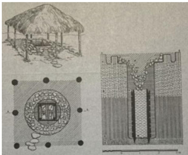
Obr. 7: Nálezová situace velkomoravské studny ze Starého Města s rekonstrukcí pravděpodobného vzhledu přístřešku, podle V. Hrubého. (GALUŠKA, Luděk. Slované – doteky předků: O životě na Moravě 6.–10. století . Brno: Moravské zemské muzeum, 2004, s. 19.)
